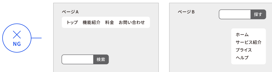
図3.19 ページによってグローバルナビゲーションの位置が異なると、ページ切り替えの度にナビゲーションを探さなくてはならない。また、ナビゲーション内の表記がページごとに揺れていると迷わせることになる
