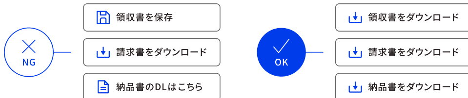
図3.20 NG例はいずれもPDFをダウンロードするボタンだが、アイコンや表記に一貫性がない
